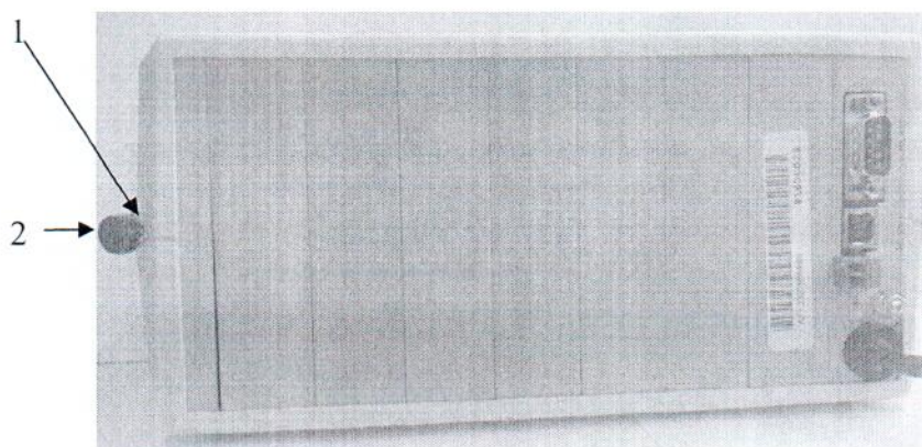
Рисунок 2 – Схема пломбировки от несанкционированного доступа, обозначение места нанесения знака поверки комплексов поверочных «ВЗЛЕТ КПИ»
