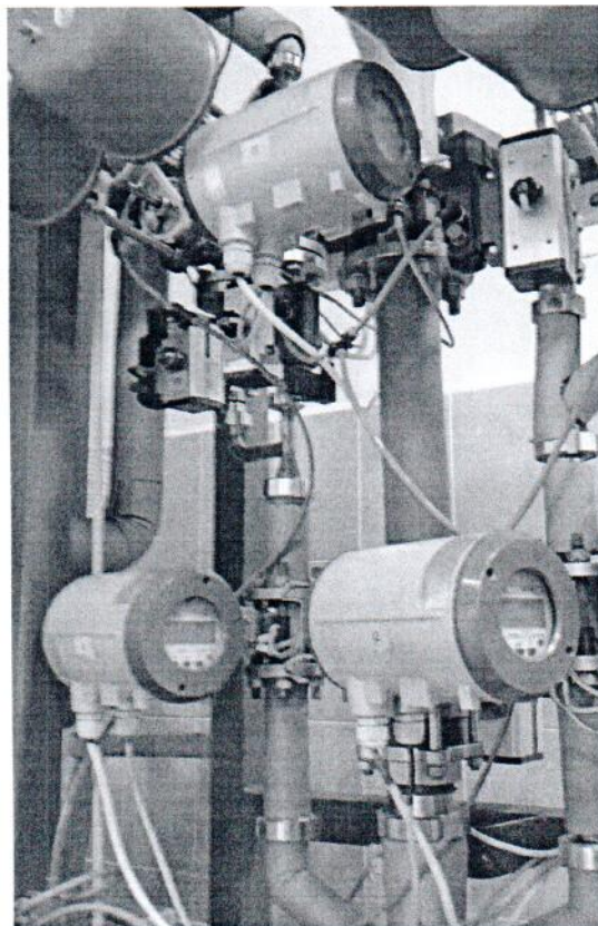
Рисунок 2 – Фотография блока индикации расхода
