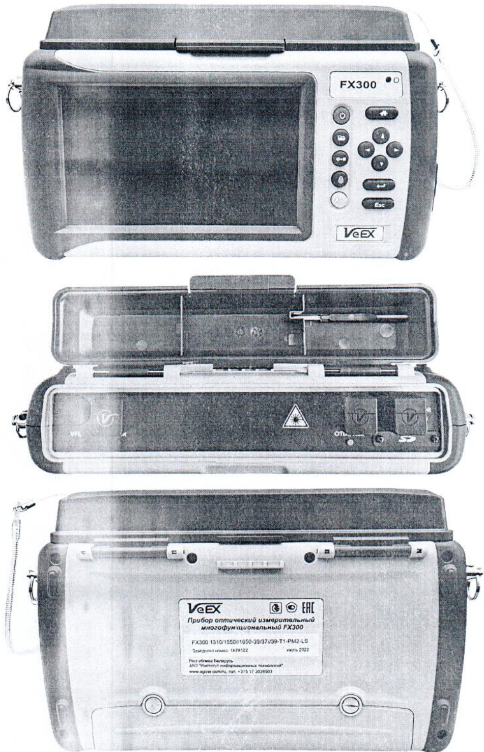
Рисунок 1.1 – Фотографии общего вида прибора FX300 (изображение носит иллюстративный характер)
