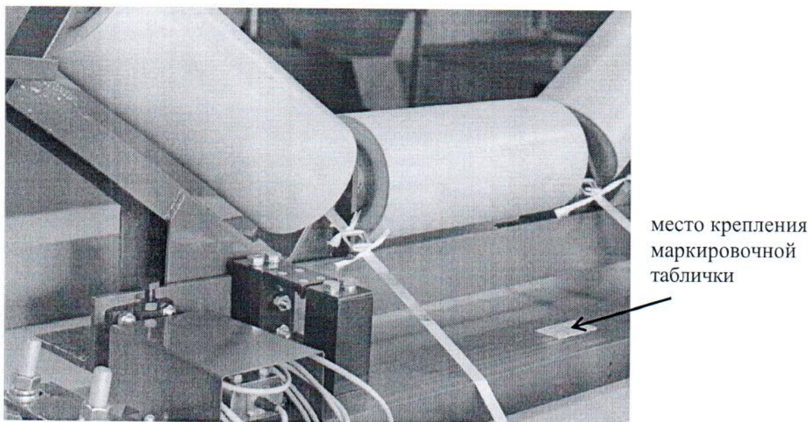
Рисунок 1 - Общий вид весов конвейерных ВК-М
