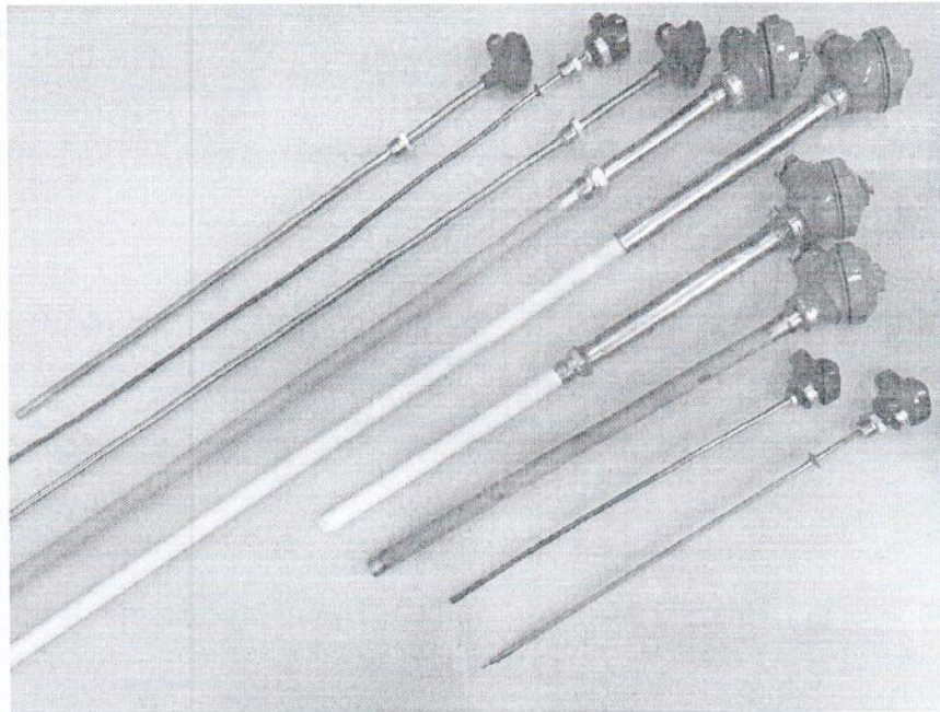
Рисунок 1.1 – Фотография общего вида преобразователей термоэлектрических ТХА(К)-1199, ТХК(Л)-1199, ТЖК(Ж)-1199, ТНН(Н)-1199, ТПП(С)-1199, ТПП(Р)-1199, ТПР(В)-1199 в исполнениях с клеммной головкой (изображение носит иллюстративный характер)
