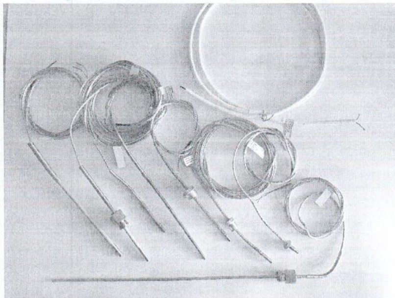
Рисунок 1.1 – Фотография общего вида преобразователей термоэлектрических ТХА(К)-1199, ТХК(Л)-1199, ТЖК(Ж)-1199, ТНН(Н)-1199, ТПП(С)-1199, ТПП(Р)-1199, ТПР(В)-1199 в исполнениях без клеммной головки (изображение носит иллюстративный характер)
