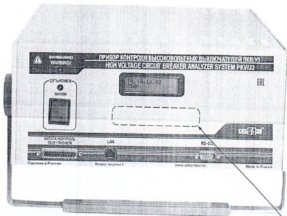
Рисунок 1 - Общий вид средства измерений 1 - место для нанесения знака поверки
