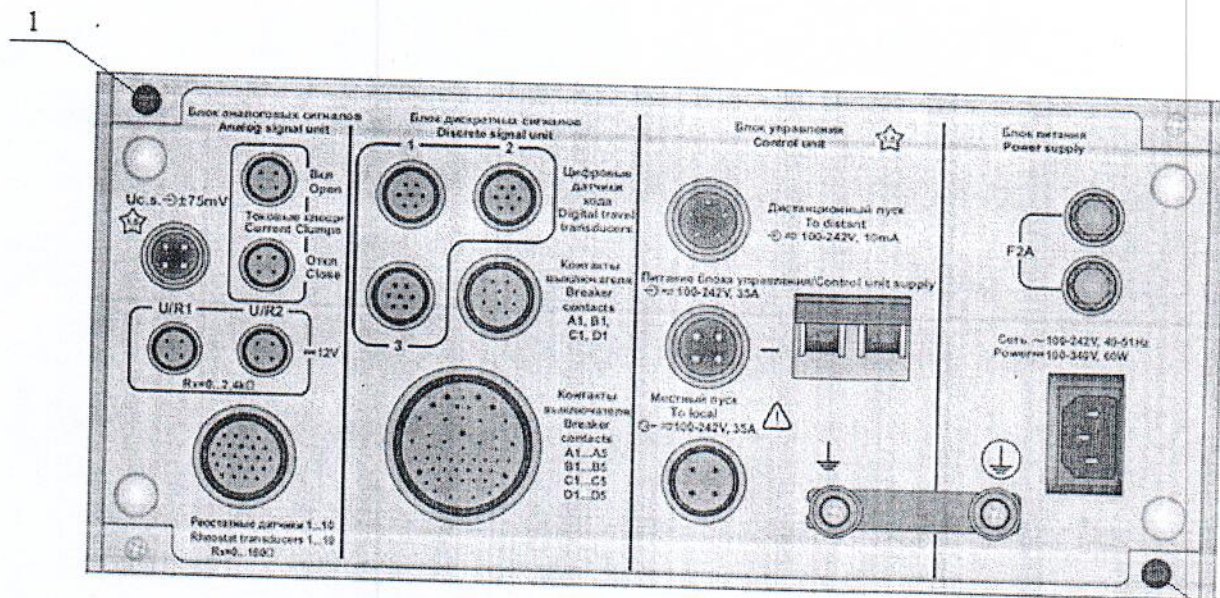
Рисунок 2 - Схема пломбировки от несанкционированного доступа (задняя панель измерительного блока ПКВ/У3.0) 1 - места нанесения оттисков пломб
