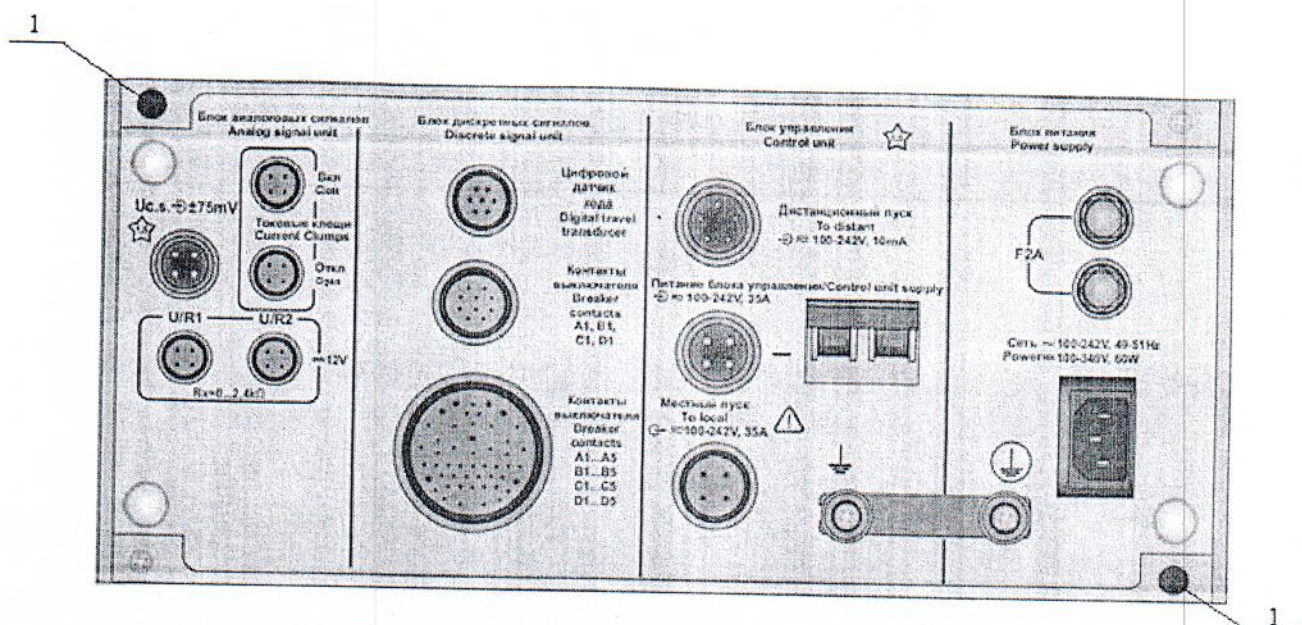
Рисунок 3 - Схема пломбировки от несанкционированного доступа (задняя панель измерительного блока ПКВ/УЗ.1)
