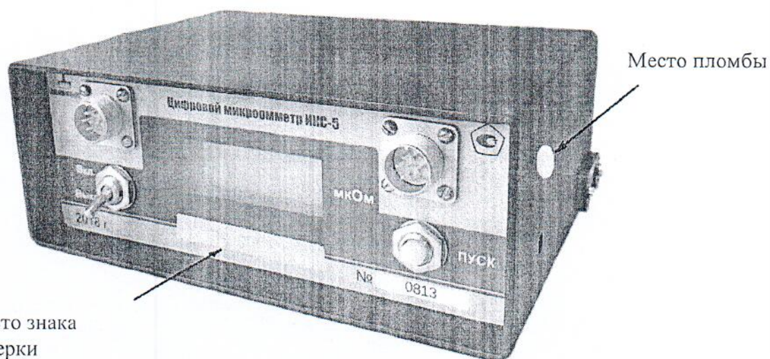
Рисунок 3 – Внешний вид микроомметра ИКС-5 исполнение 2
