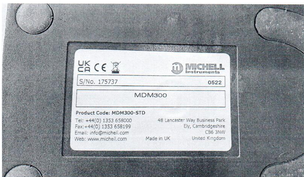
Рисунок 1.2 – Маркировка гигрометра MDM300 № 175737
