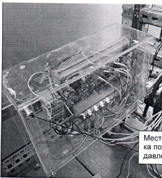
Рисунок 3.4 – Места пломбировки модуля нормализации частотных сигналов ТВА 8-6
