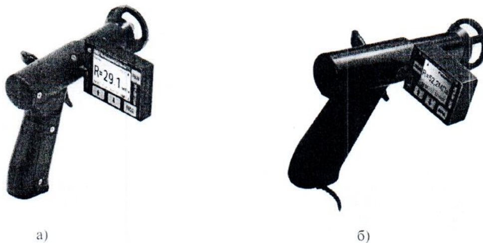
Рисунок 2 а, б – Общий вид измерителя прочности бетона мод. ИПС-МГ4.04
