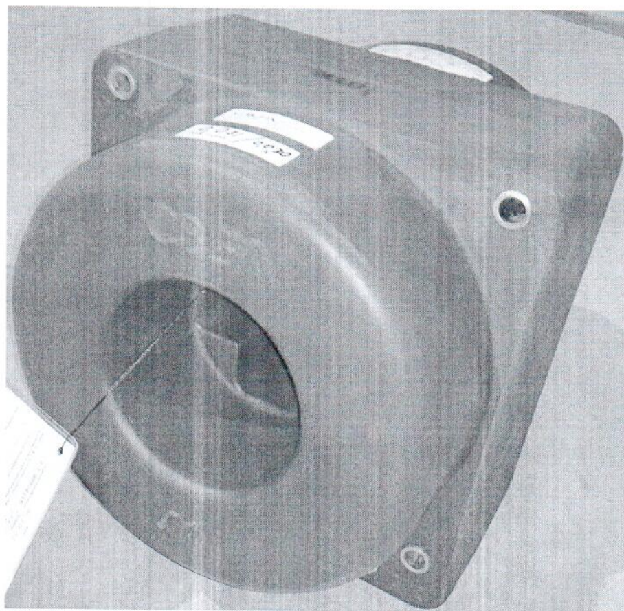
Рисунок 2 - Общий вид трансформаторов тока ТШЛ-СВЭЛ-10
