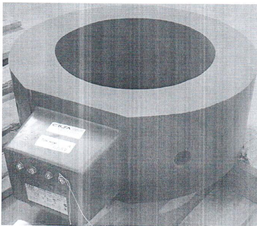
Рисунок 3 - Общий вид трансформаторов тока ТШЛ-СВЭЛ-20
