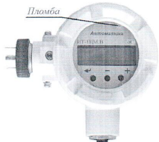
б) Лицевая фальшпанель преобразователей ИТ-1Ц.В(-Ех), ИТ-2Ц.В, ИТ-1ЦМ.В(-Ех), ИТ-2ЦМ.В
