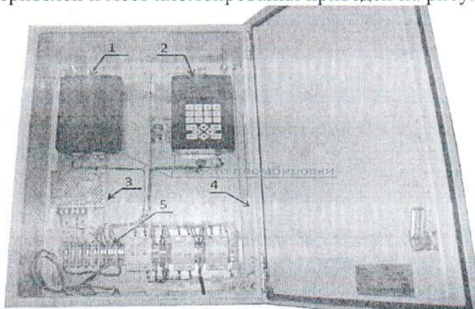
Рисунок 1 - Общий вид блока измерительного ИС-14.М 1 - вычислитель; 2 - контроллер ИС-14.М; 3 - источник питания; 4 - лампа освещения; 5 - клеммная колодка
