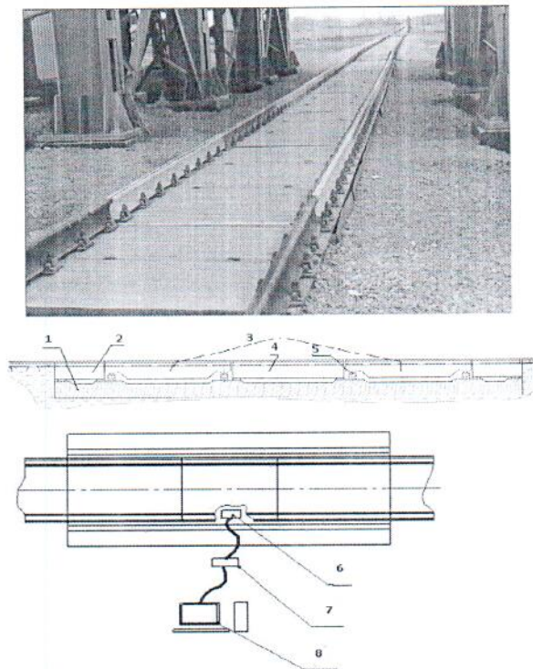
Рисунок 1 – Общий вид ГПУ и схематичное изображение весов (1 – железобетонный фундамент; 2 – въездная секция; 3 – секция ГПУ, 4 – промежуточная секция; 5 – датчик; 6 – ДП-4 (ДП-8); 7 – адаптер интерфейсный; 8 – ПК)
