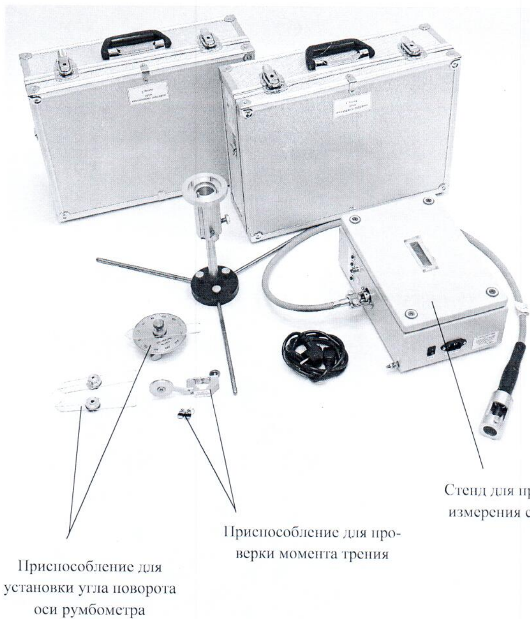
Рисунок 1.1 – Фотография общего вида комплекса поверочного КИ – 01
