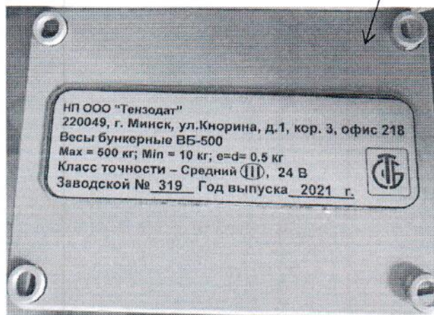
Рисунок 2.1 – Фотография с указанием места нанесения знака поверки (наклейки) на преобразователь тензометрический ПТН-1
