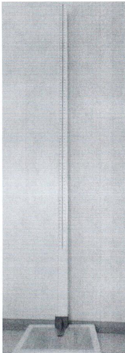
Рисунок 1.1 – Фотография общего вида ростомера медицинского РМ-1П № 6893
