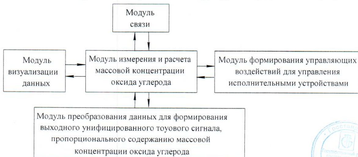
Рисунок 3 - Структура ПО
