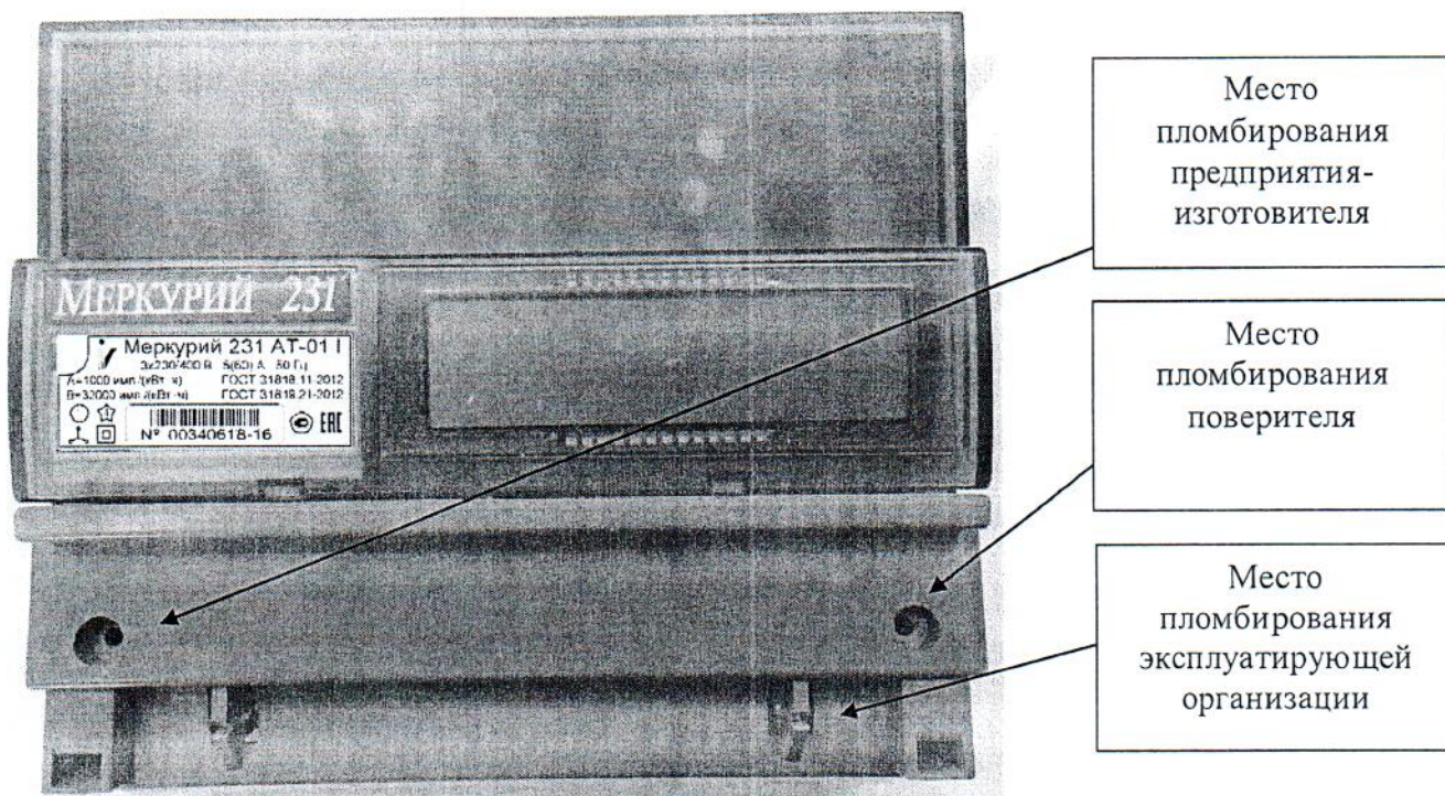
Рисунок 3 – Общий вид счетчиков «Mercury 231 AT-0X», «Mercury 231 AT-0X» с указанием мест пломбирования и нанесения знака поверки
