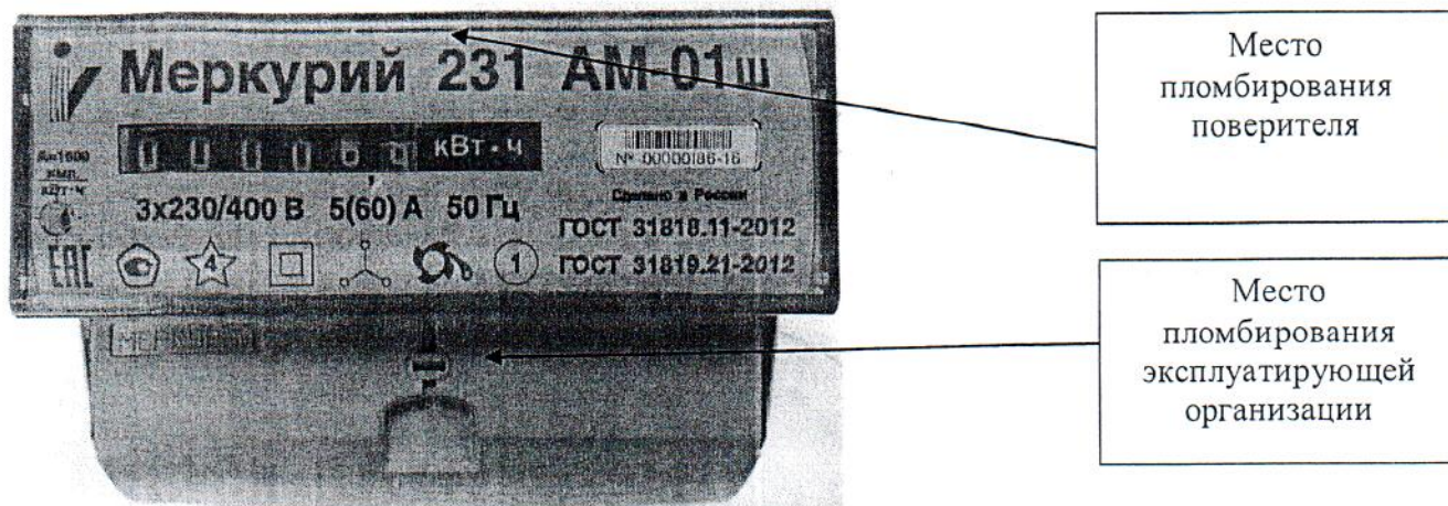
Рисунок 2 – Общий вид счетчиков «Mercury 231 AM-0Xш», «Mercury 231 AM-0Xш» с указанием мест пломбирования и нанесения знака поверки
