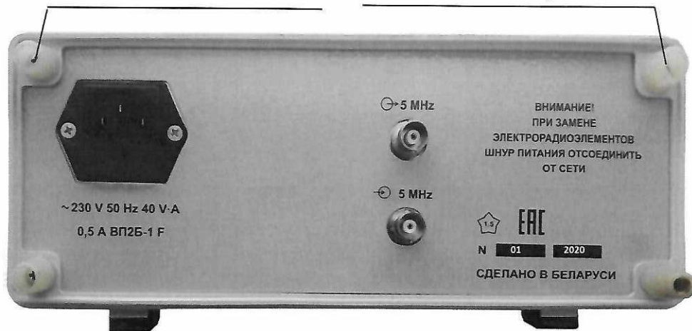
Рисунок 2.3 – Место пломбирования ОТК и нанесения оттиска знака поверки (вид частотомера сзади)
