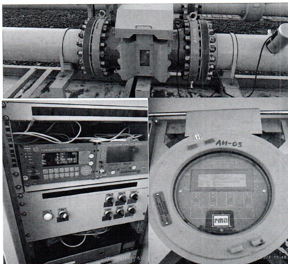
Рисунок 1.1 – Фотография общего вида ИС УУГ
