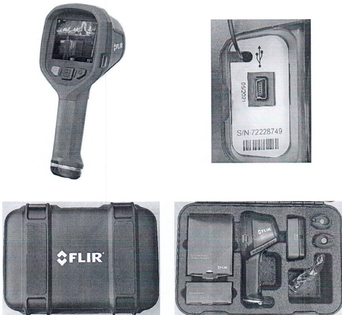
Рисунок 1.1 – Общий вид и маркировка камеры тепловизионной FLIR K65 № 72228749
