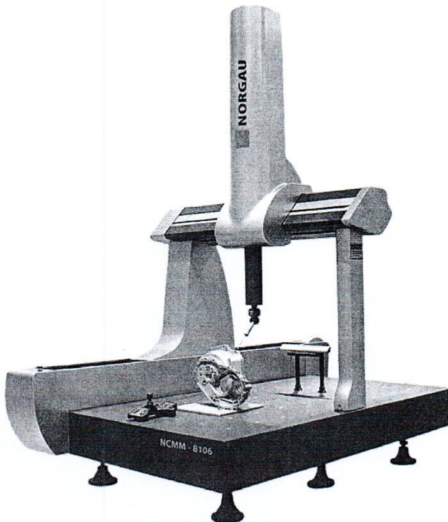
Рисунок 1 - Общий вид машин координатно-измерительных NORG AU серии NCMM.
