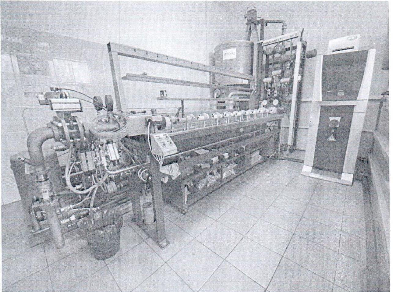
Рисунок 1 – Фотография общего вида установки поверочной расходомерной Prematest 50 Z № 001/2005
