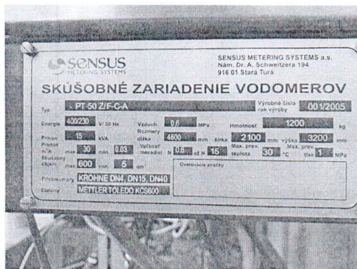
Рисунок 2 – Фотография маркировки установки поверочной расходомерной Prematest 50 Z № 001/2005
