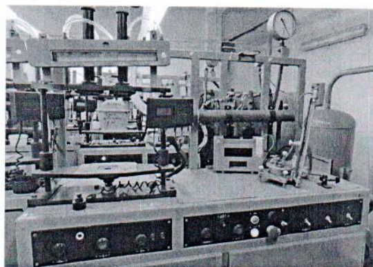
Рисунок 1.2 – Внешний вид пульта управления стенда
