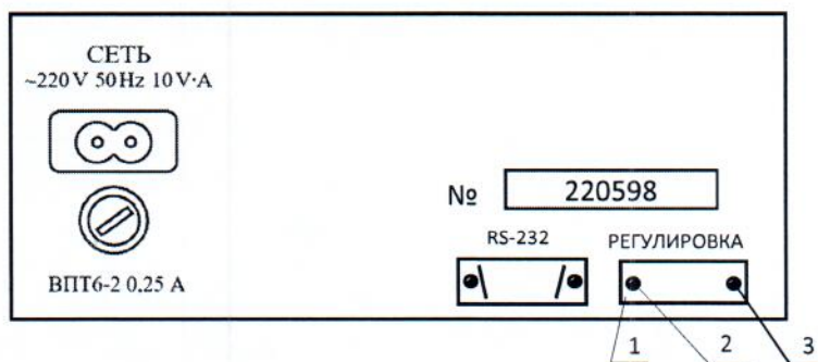
Рисунок 2.1 – Схема пломбировки от несанкционированного доступа и указание мест для нанесения отиска клейма и знака поверки на верхнюю часть корпуса приборов
