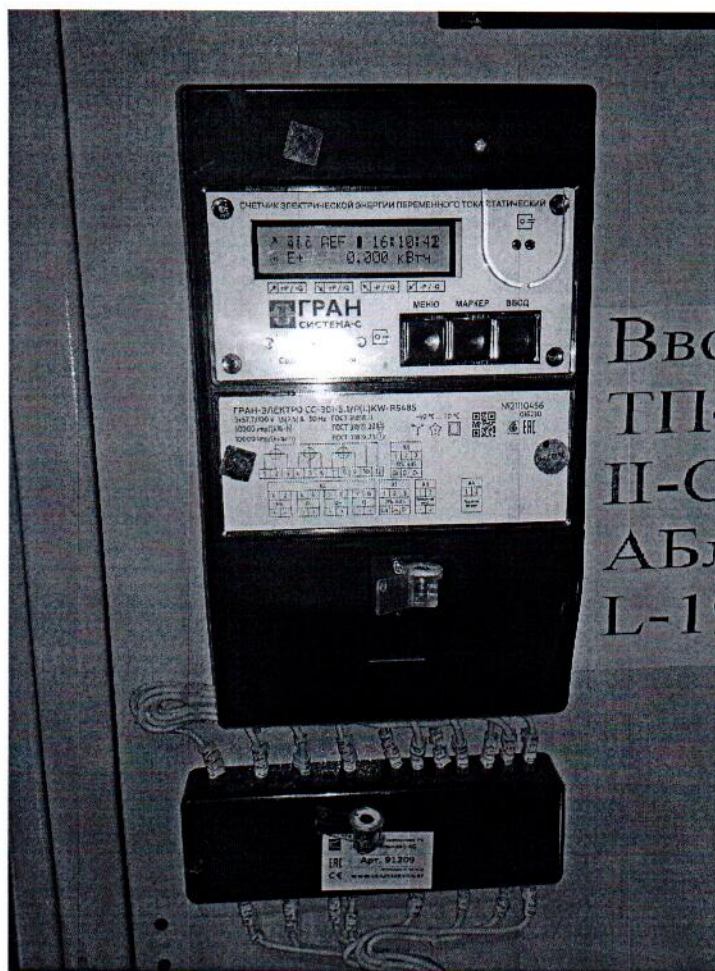
Рисунок 2 – Фотография компонентов измерительного канала АСКУЭ при применении счетчика электрической энергии «Гран-Электро СС-301»
