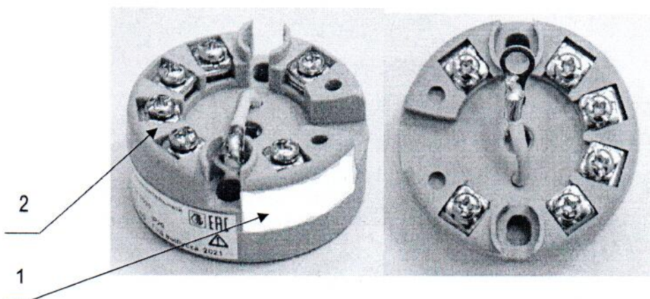
Рисунок 1.1 – Общий вид преобразователей сигналов CS-A, CS-AEx
