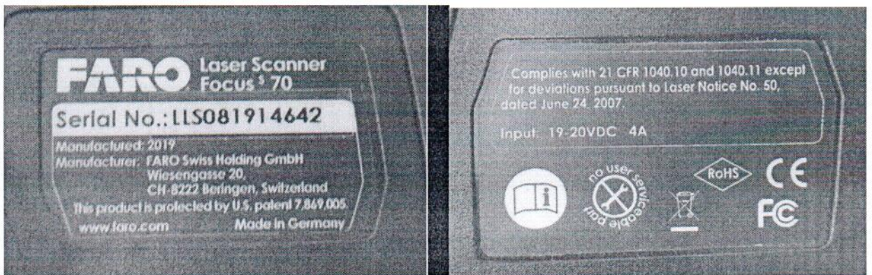
Рисунок 1.2 – Фотография маркировки лазерного сканера FARO Focus S70 № LLS081914642
