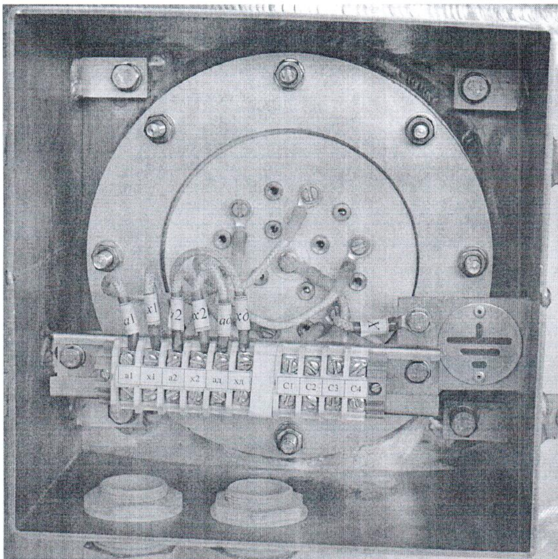
Рисунок 2 - Клеммная коробка
