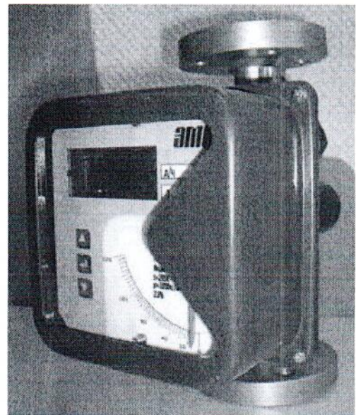
Рисунок 1.5 – Общий вид ротаметра ЭМИС-МЕТА 215, DN 15 с дополнительным считыванием показаний по ЖК дисплею
