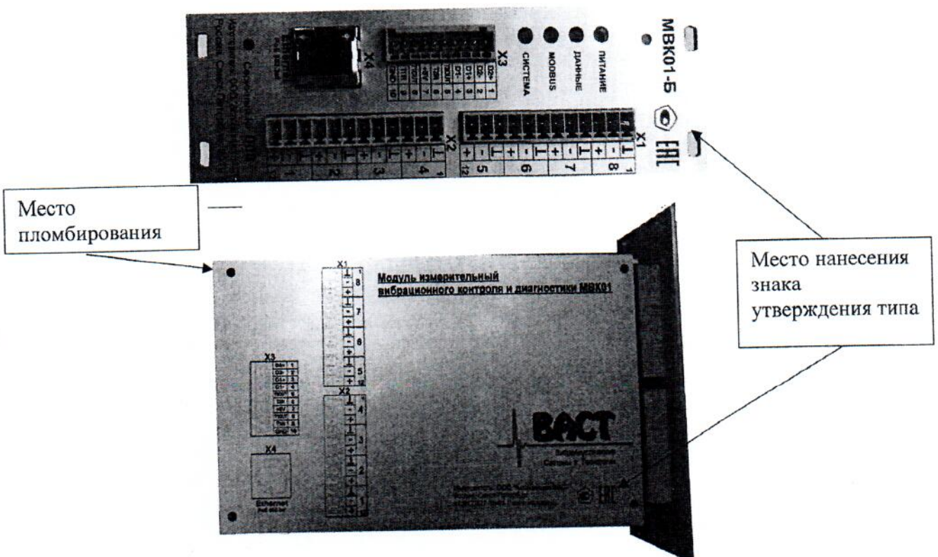
Рисунок 2 - Общий вид, место нанесения знака утверждения типа и место пломбирования от несанкционированного доступа модулей измерительных вибрационного контроля и диагностики MBK01-Б
