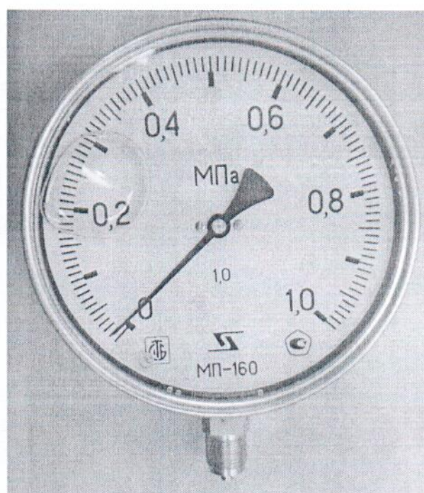
Манометр показывающий МП-160 с жидкостным наполнением
