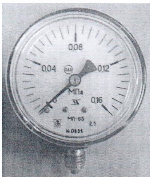
Манометр показывающий МП-63
