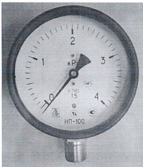
Напоромер показывающий НП-100
