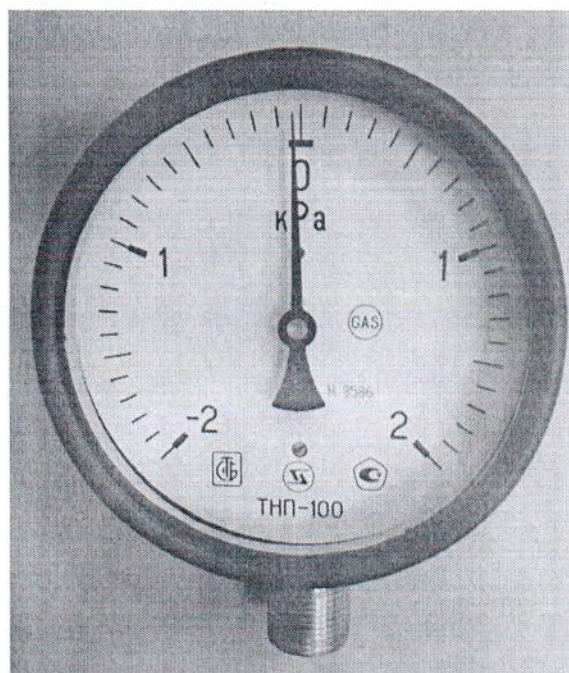
Тягонапоромер показывающий ТНП-100
