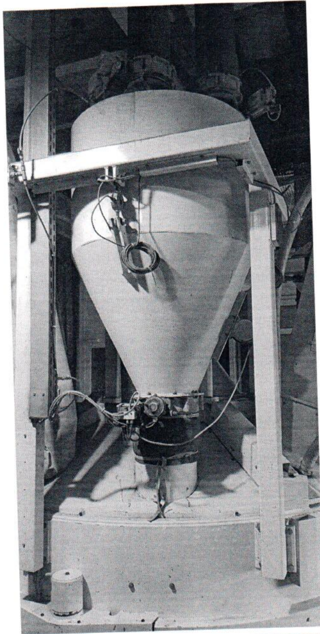
Рисунок 1.1 – Внешний вид дозатора весового дискретного действия цемента ДВДДц-1000 №11702658_5
