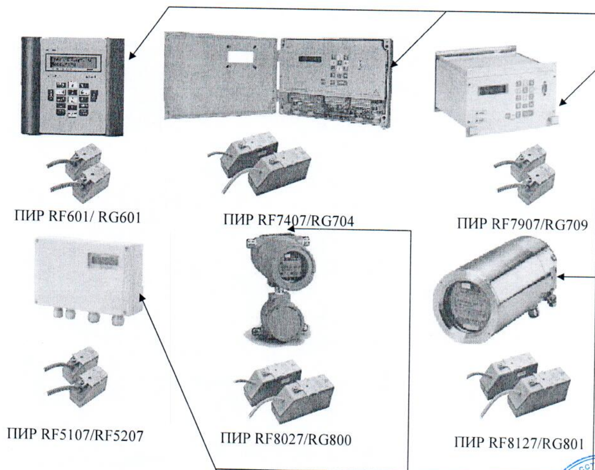
Рисунок 1 – Внешний вид расходомеров ПИР
