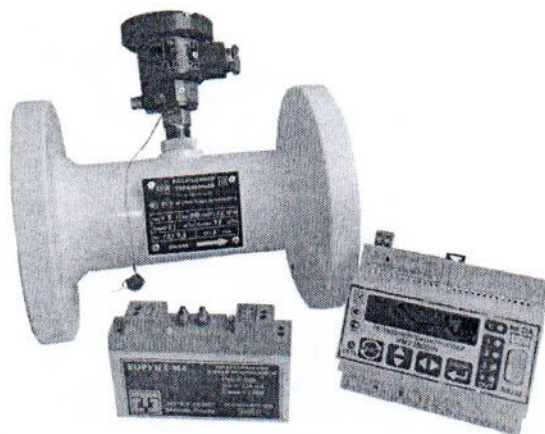
Рисунок 2 – Общий вид счетчика в комплекте с ПР
