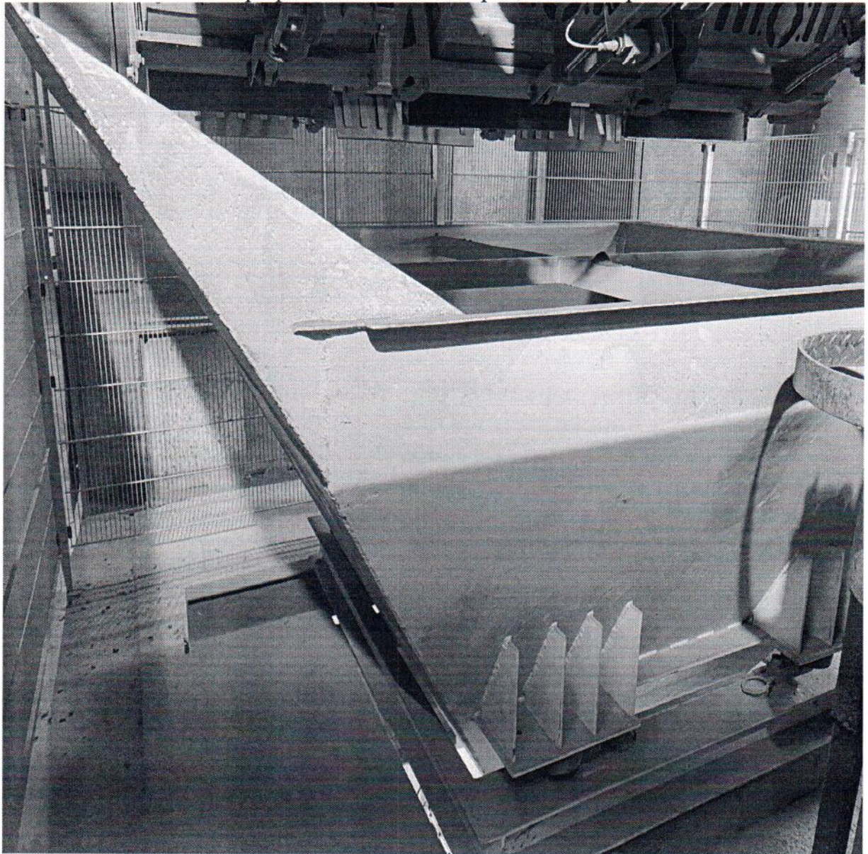
Рисунок 1.1 – Внешний вид дозатора весового дискретного действия инертных материалов ДВДДи-3000 №11702658_1
