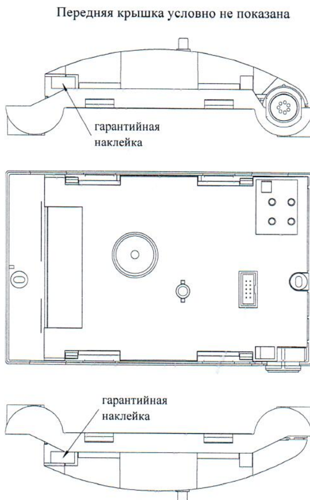
Рисунок 2 – Схема пломбировки сигнализаторов от несанкционированного доступа и обозначение мест для нанесения гарантийных наклеек
