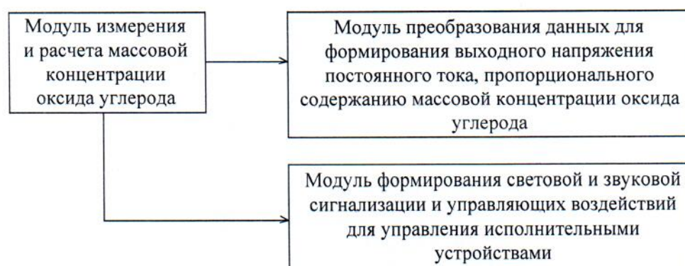
Рисунок 3 – Структура ПО
