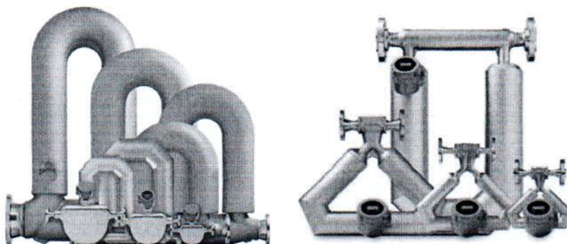
Рисунок 1.1 Общий вид первичных преобразователей моделей CMF с электронным преобразователем модели 2400
