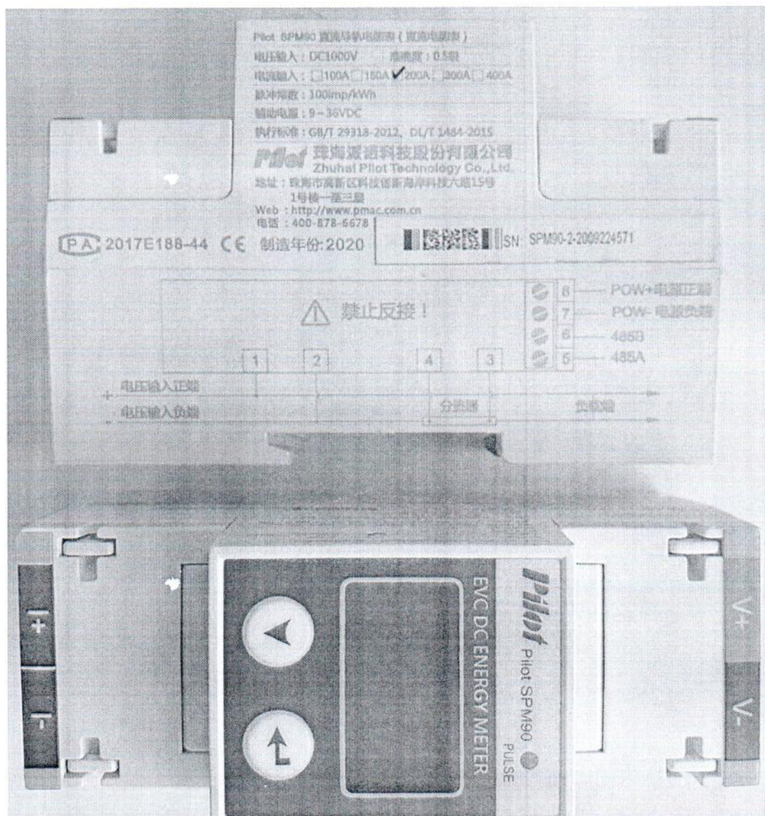
Рисунок 1.1 – Внешний вид счетчика SPM90 зав. № SPM90-2-2009224571
