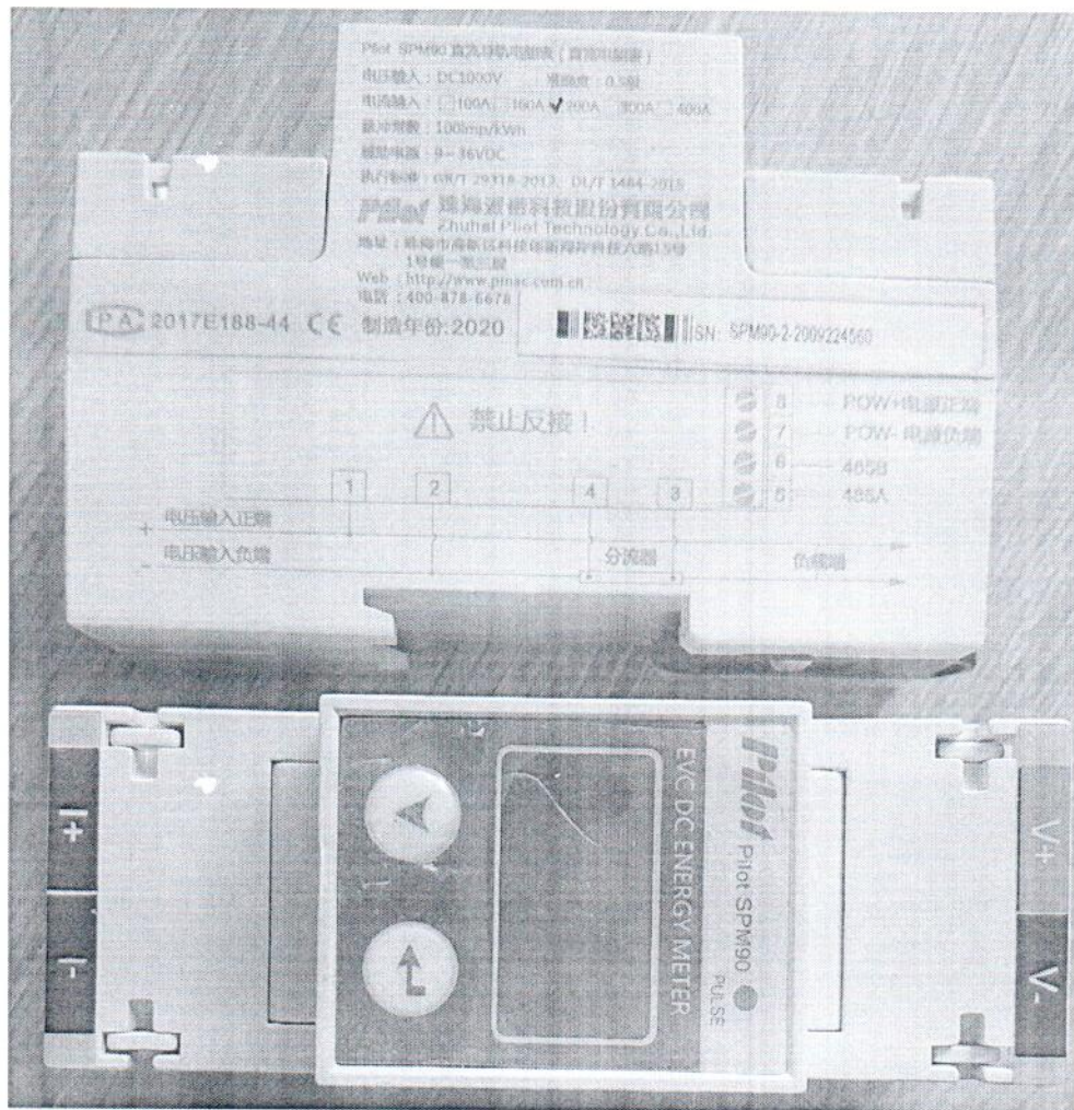
Рисунок 1.1 – Внешний вид счетчика SPM90 зав. № SPM90-2-2009224560
