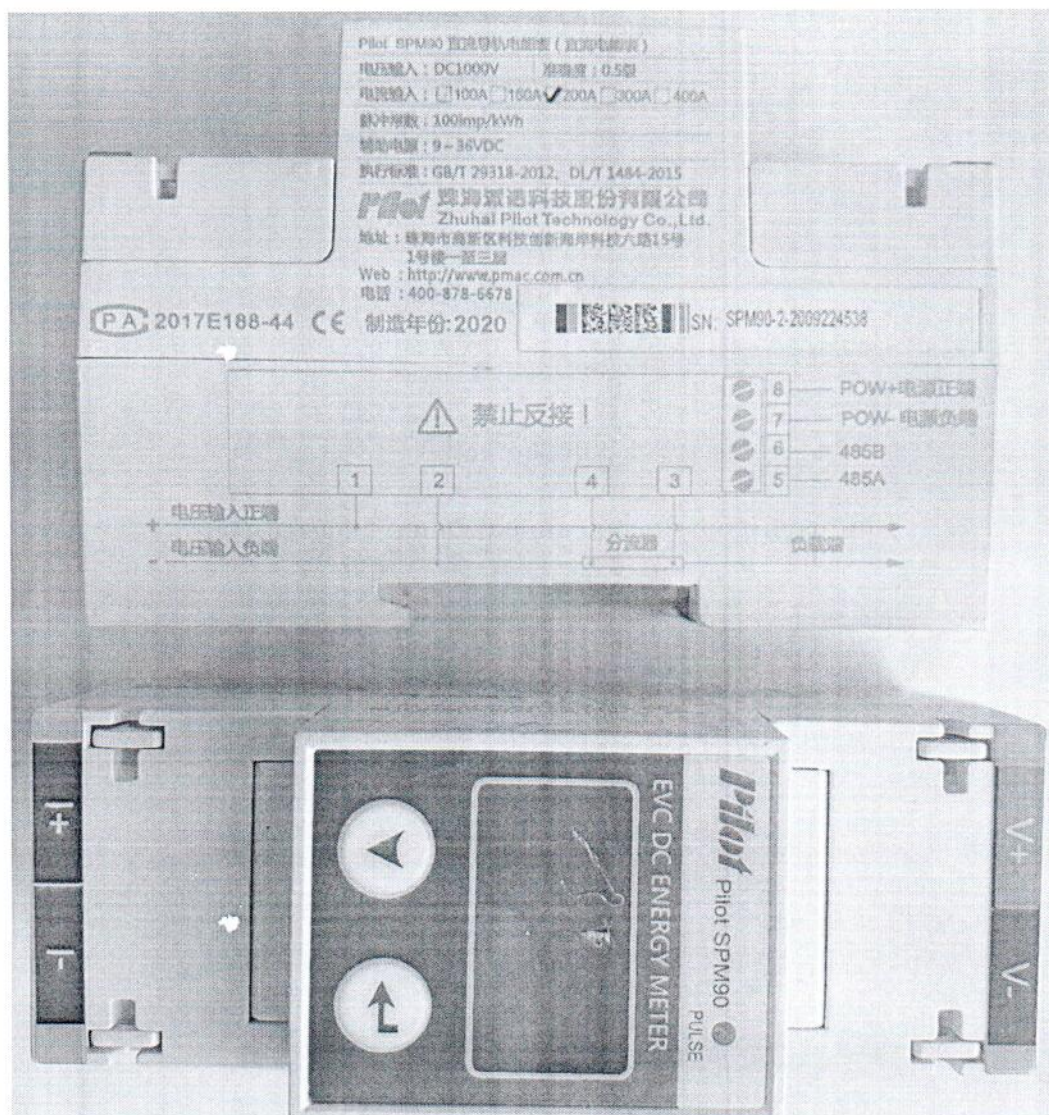
Рисунок 1.1 – Внешний вид счетчика SPM90 зав. № SPM90-2-2009224538
