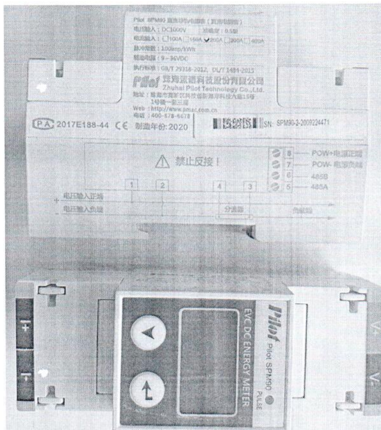
Рисунок 1.1 – Внешний вид счетчика SPM90 зав. № SPM90-2-2009224471
