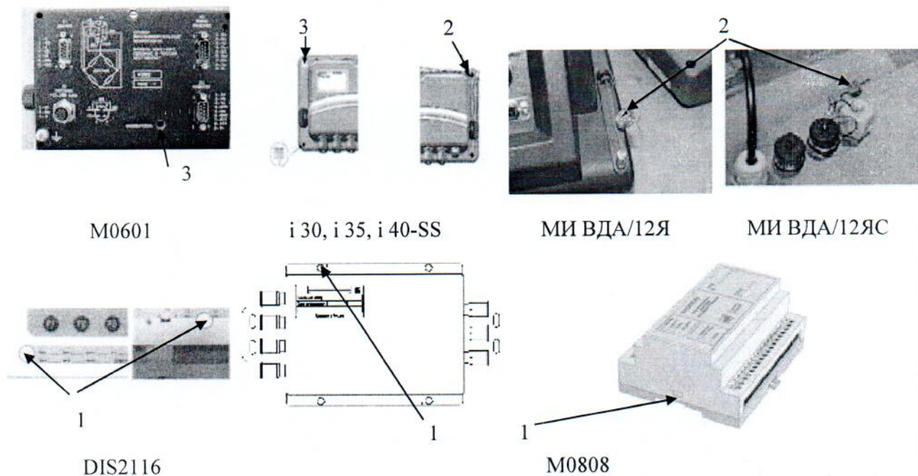
Рисунок 5 – Схема пломбировки от несанкционированного доступа(1–пломба в виде разрушаемой наклейки, 2–свинцовая или пластиковая пломба, 3–мастичная пломба)
