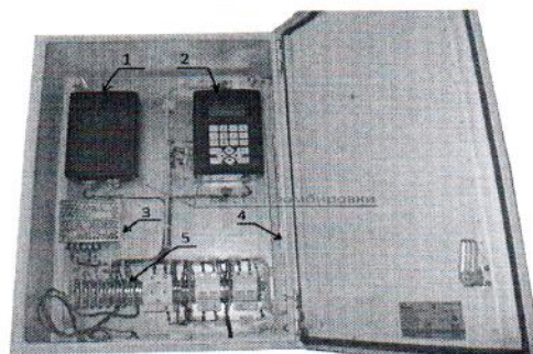
Рисунок 1 – Общий вид блока измерительного ИС-14.М 1 – вычислитель; 2 – контроллер ИС-14.М; 3 – источник питания; 4 – лампа освещения; 5 – клеммная колодка
