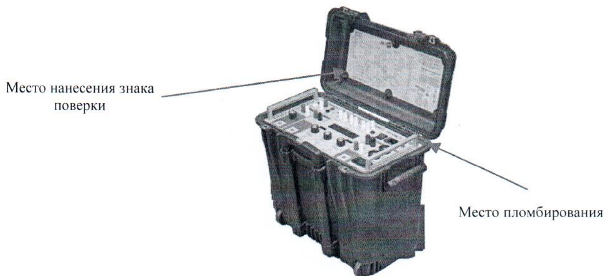
Рисунок 1 – Общий вид устройств, места пломбирования и нанесения знака поверки
