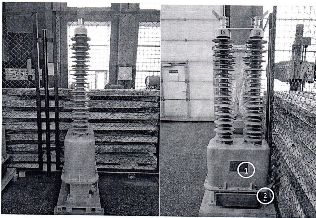
Рисунок 1 - Фотографии общего вида со схемой нанесения знака поверки и места пломбировки 1 - место нанесения знака поверки, 2 - место пломбировки от несанкционированного доступа
