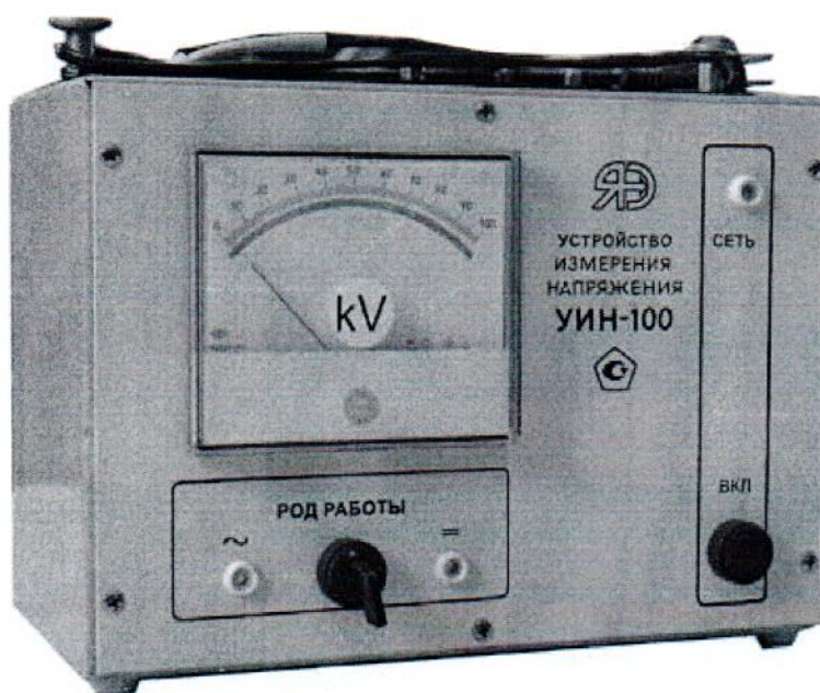
Рисунок 2 – Общий вид устройство измерения напряжения УИН-100
