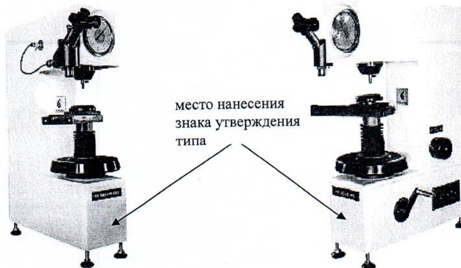
Рисунок 2 – Общий вид твердомеров УТ 5021МС Tochline
