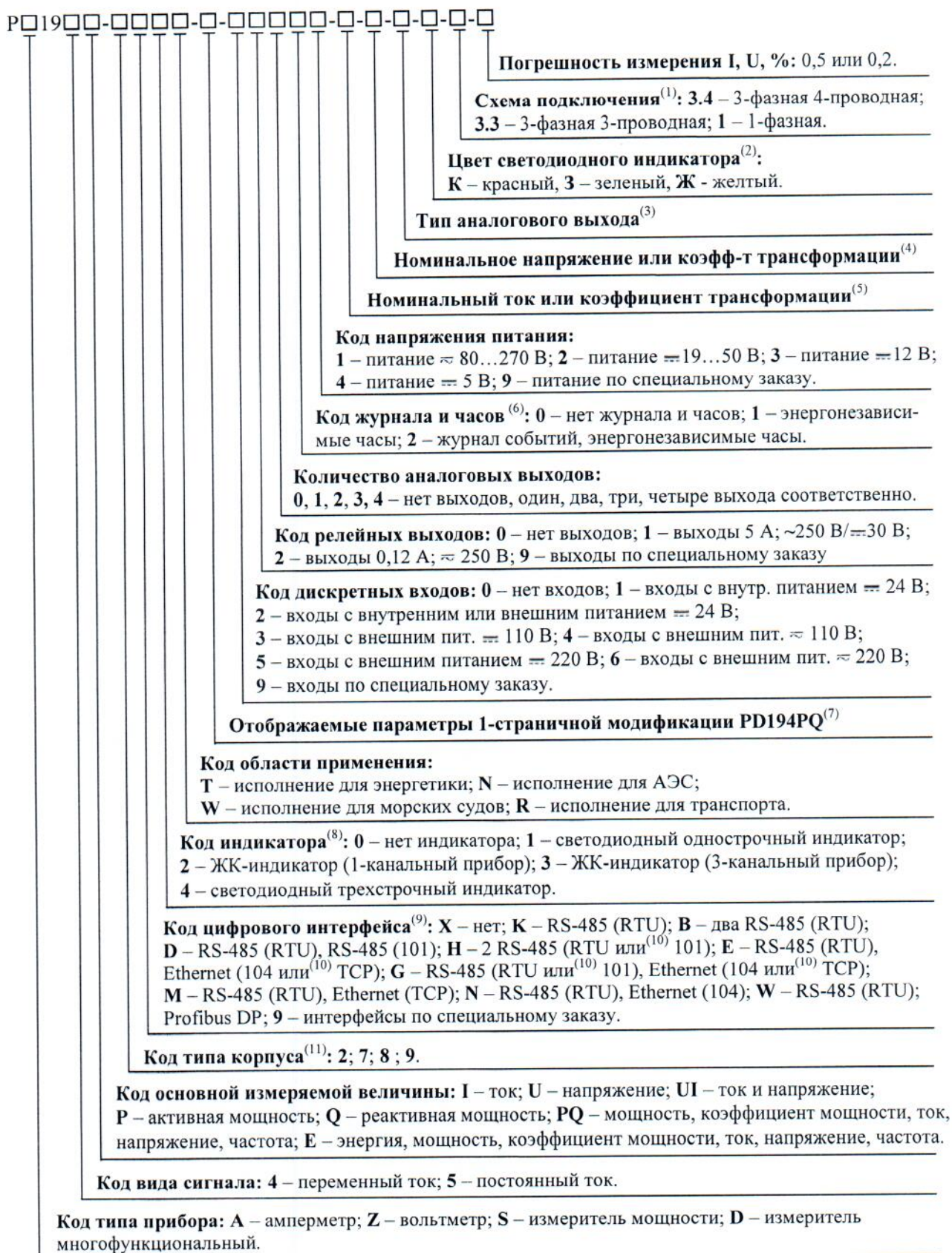
Рисунок 1 – Структура условного обозначения модификаций прибора
